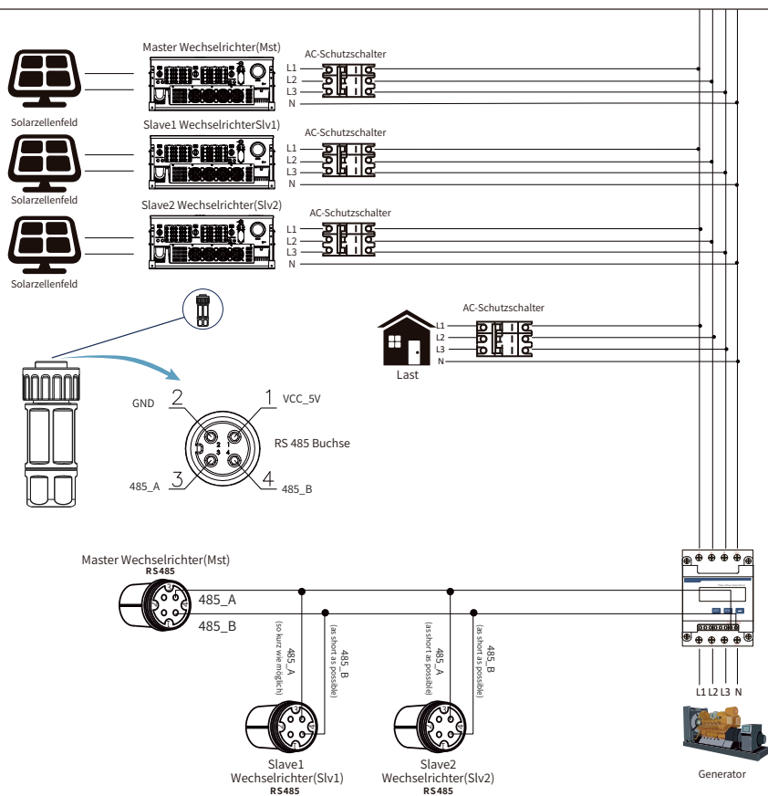
Abb. 7.29 CHINT Anschlussplan (Die Durchleitungstabelle)
