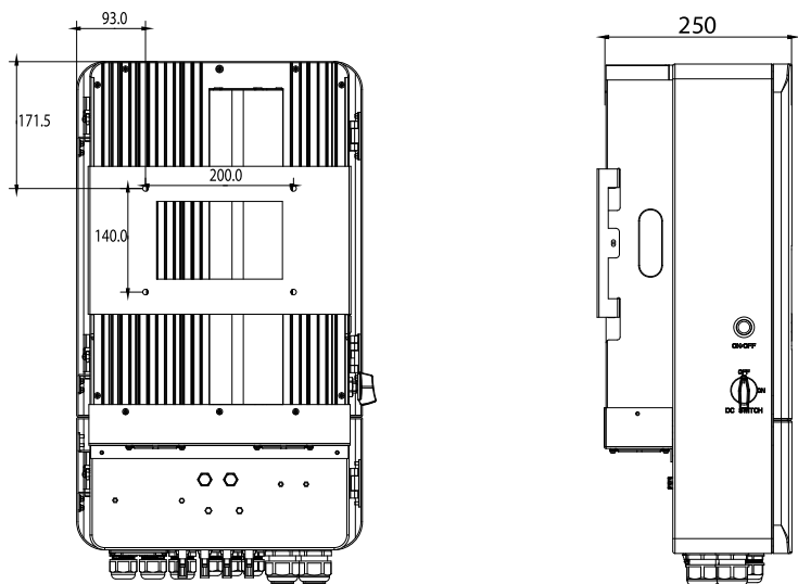
Abmessungen des Wechselrichters
