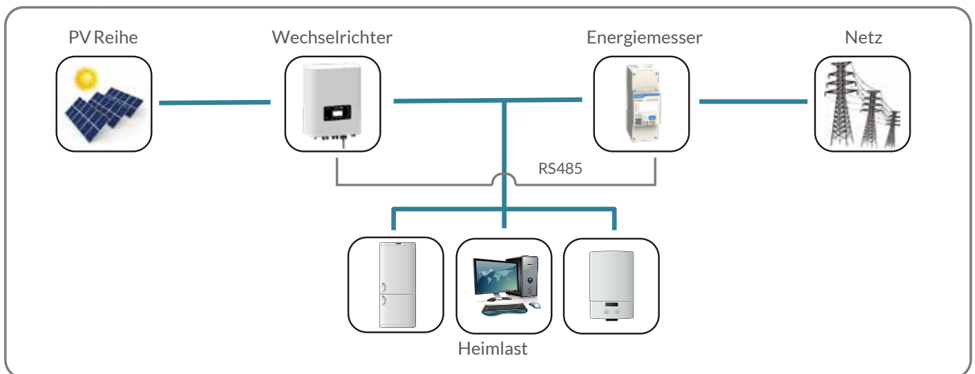
Typisches Anwendungsdiagramm
