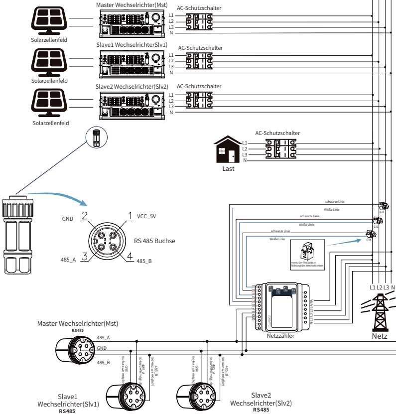
Abb. 7.23 Anschlussplan (Dreiphasenstrom)
