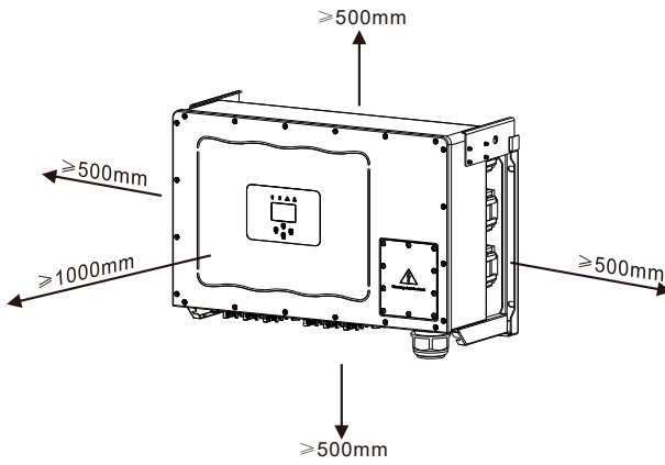
Abb. 4.3 Einbaulücke
