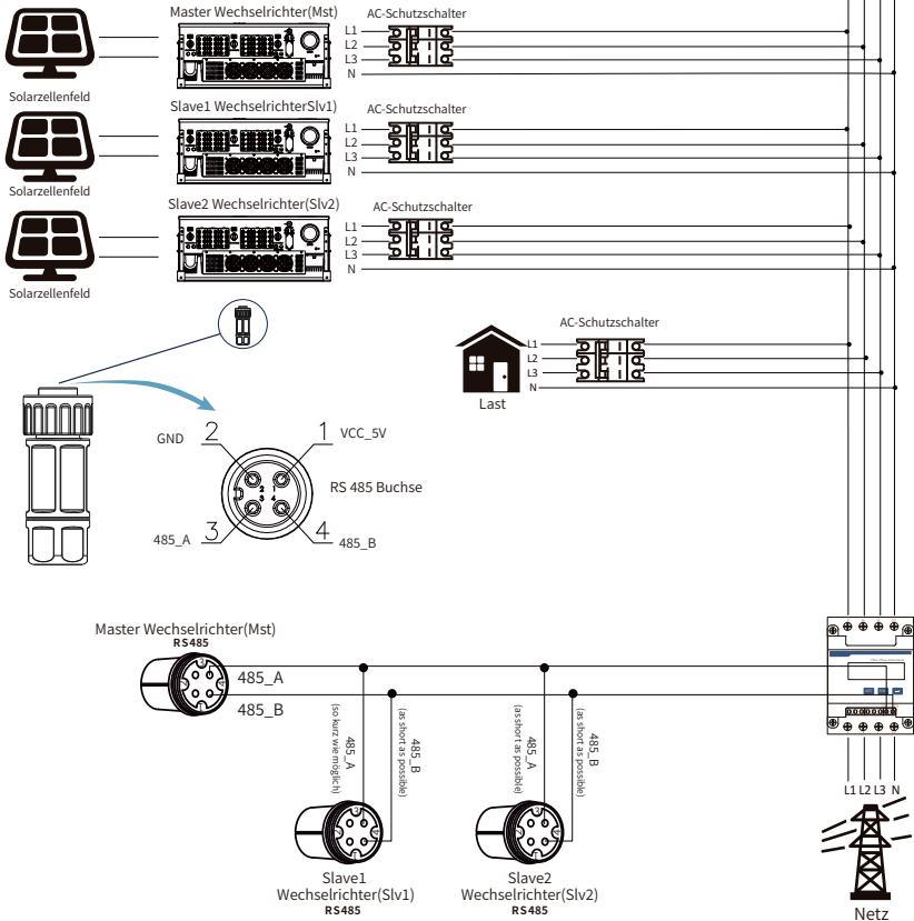
Abb. 7.27 CHINT Anschlussplan (Die Durchleitungstabelle)
