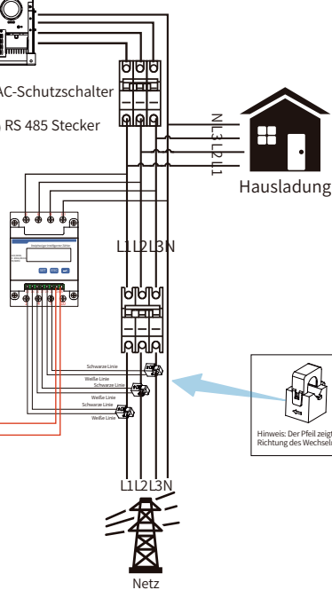
Abb. 7.14 Anschlussplan des CHINT-Zählers
