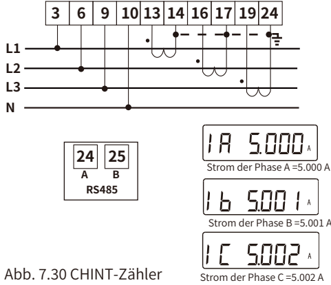
Abb. 7.30 CHINT-Zähler
