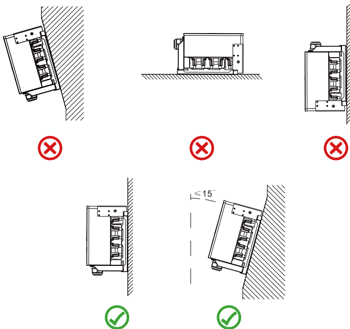
Abb. 4.2 Einbauwinkel
