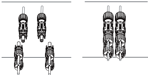
Abb. 3.6 DC-Eingangsanschluss
